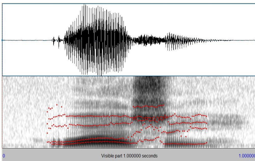
Spektrogram 6: Contoh kehadiran tempoh frikasi bunyi Melayu Arab /s/ tak bersuara di tengah kata
