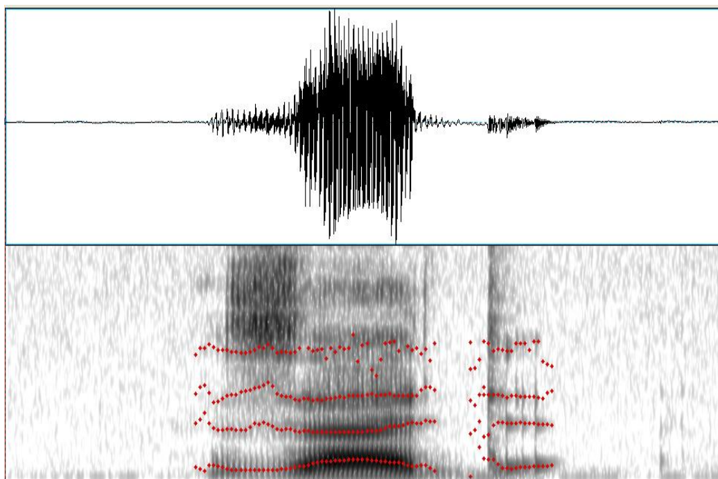
Spektrogram 3: Contoh kehadiran tempoh frikasi bunyi Melayu Arab /ج/ di awal kata
