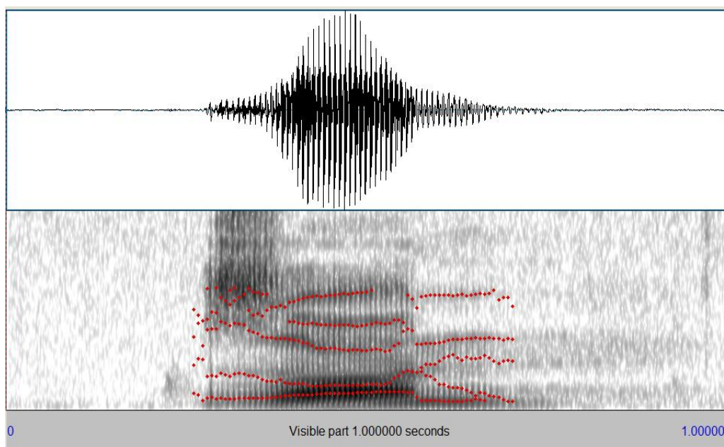
Spektrogram 7: Contoh kehadiran tempoh frikasi bunyi Melayu Arab /z s / di awal kata
