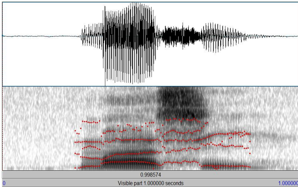
Spektogram 2: Contoh kehadiran tempoh frikasi bunyi Melayu Arab /س/ di tengah kata
