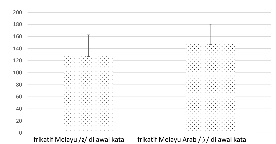
Rajah 3: Perbezaan min di antara frikatif Melayu /z/ dan frikatif Melayu Arab /ز/ di awal kata
