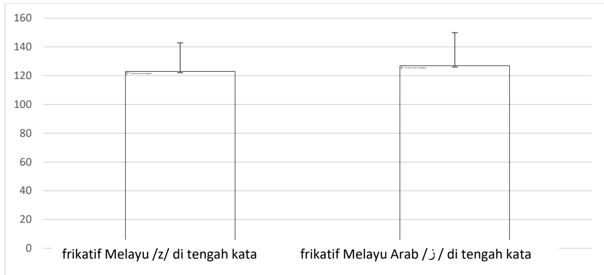
Rajah 4: Perbezaan min di antara frikatif Melayu /z/ dan frikatif Melayu Arab /ز/ di tengah kata
