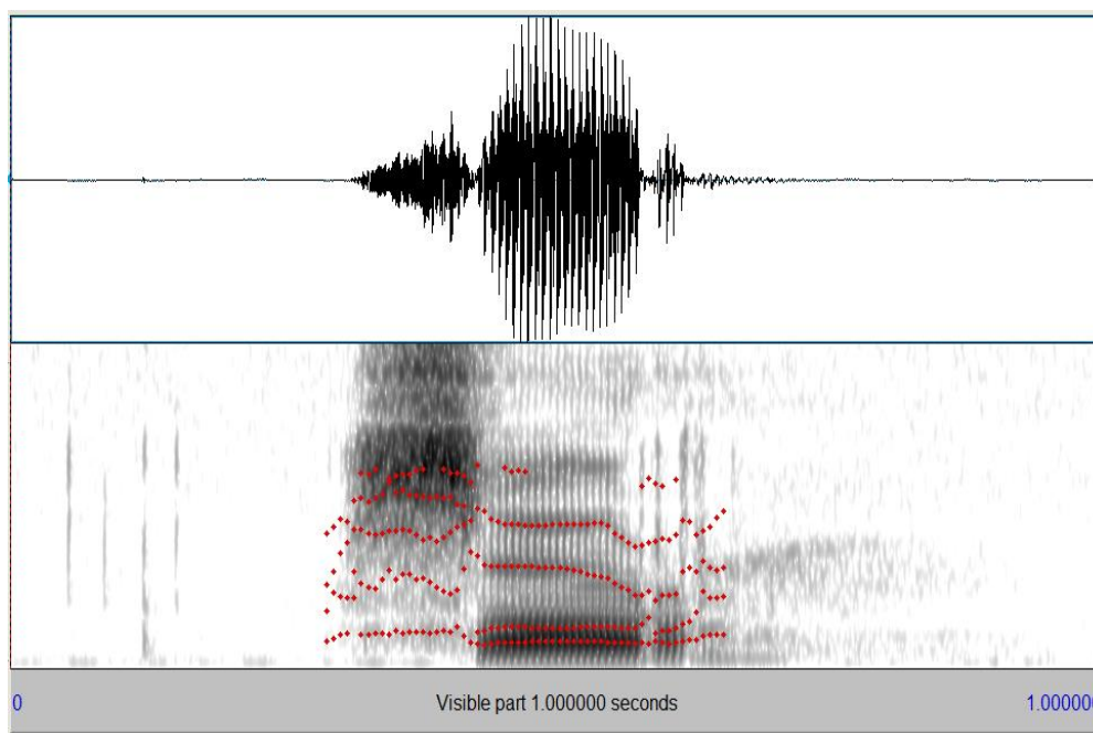
Spektrogram 5: Contoh kehadiran tempoh frikasi bunyi Melayu Arab /sʰ/ tak bersuara di awal kata
